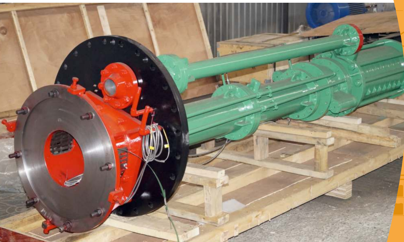
Полупогружной насос для нефтехимии НХТ 200/450 в г. Красноярск
