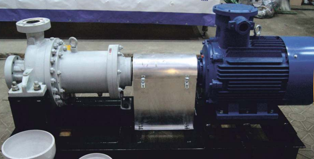
Насосный агрегат ГММ 5/300-НГС с эл.двигателем ВА200М2 в г. Москва
